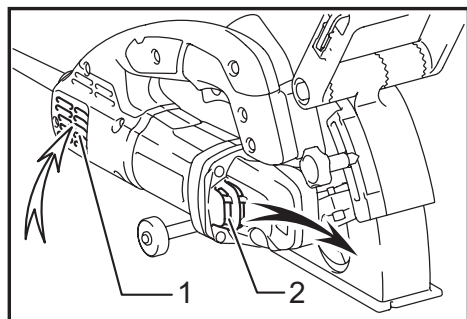
► 1. Abertura de ventilación de entrada 2. Abertura de ventilación de salida
