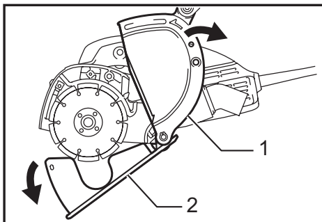
► 1. Boîtier de la lame 2. Base de l'outil
