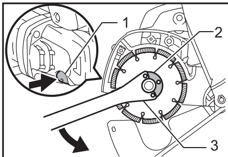
► 1. Verrouillage de l'arbre 2. Contre-écrou 3. Clé à contre-écrou
